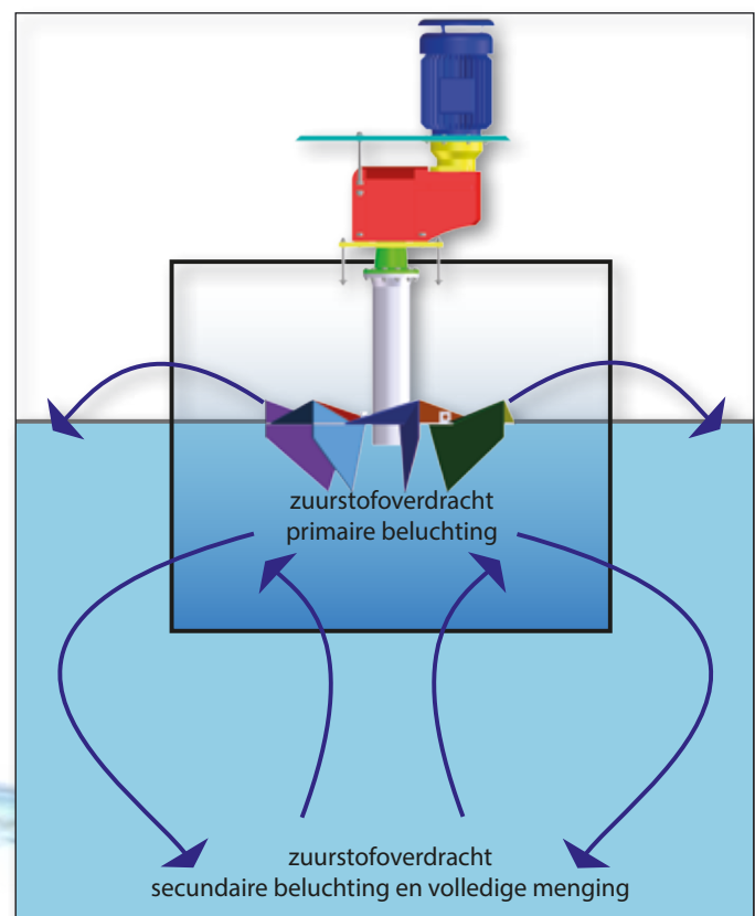
LANDY laagtoeren beluchter met axiale stroming
